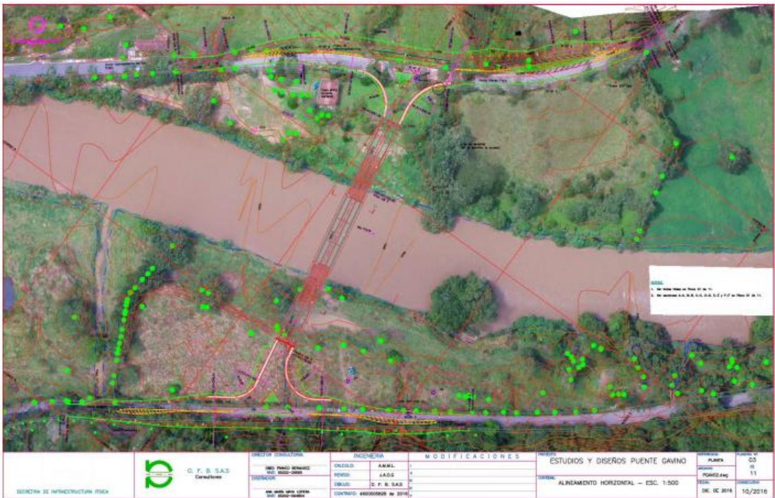
Imagen 2. Vista en planta del detalle del diseño geométrico y ubicación del puente en la zona de interés. Fuente: Estudio aportado por la Gobernación de Antioquia- secretaria de infraestructura física.
